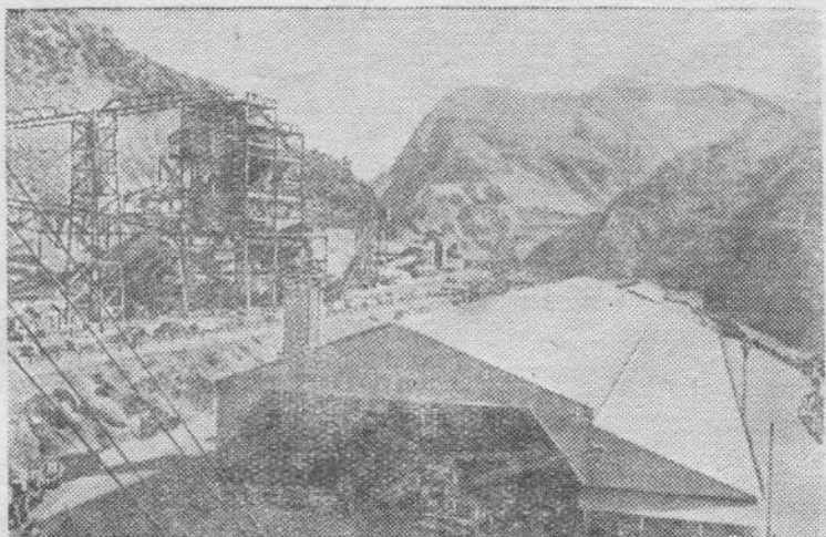
Индия. В живописных ущельях отрогов Гималаев развернулось строительство плотины и электростанции Бхакра-Наггал. На снимке: один из участков сооружения плотины. Слева — бетонный завод.
