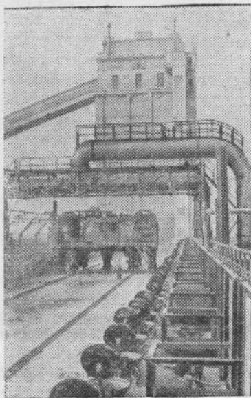
На Челябинском металлургическом заводе началась загрузка новой коксовой батареи.
