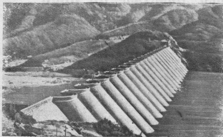
Китайская Народная Республика. Фоззалинское водохранилище на реке Бихэ (провинция Аньхуэй). Его емкость — 470 миллионов кубических метров воды.
