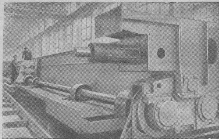
Запорожская область. Днепровский механический завод приступил к изготовлению стонных мостовых кранов. На снимке: мост стонного крана.
