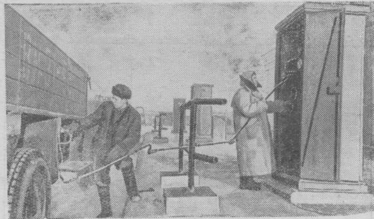
Куйбышев. В директивах XIX съезда КПСС предусмотрено широкое использование газа для бытовых нужд, применение его в качестве автомобильного топлива. В гор. Куйбышеве построена газонаполнительная станция для заправки газобаллонных автомашин. Часть автотранспорта уже переведена на газ.
