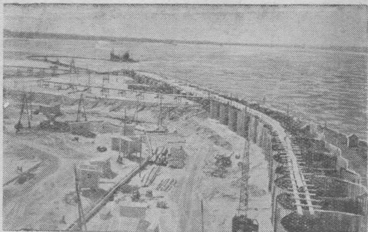
Каховский гидроузел. На участке сооружения продольной шпунтовой перемычки.
