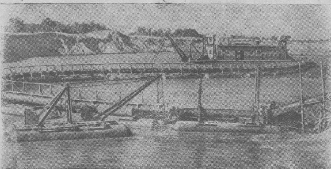
Сталинградгидрострой. Комсомольско-молодежный земснаряд 501 производит выемку грунта и намыв дамбы на трассе нижнего подходного канала к шлюзу со стороны Волги. На снимке: земснаряд 501. Прессклише ТАСС.
