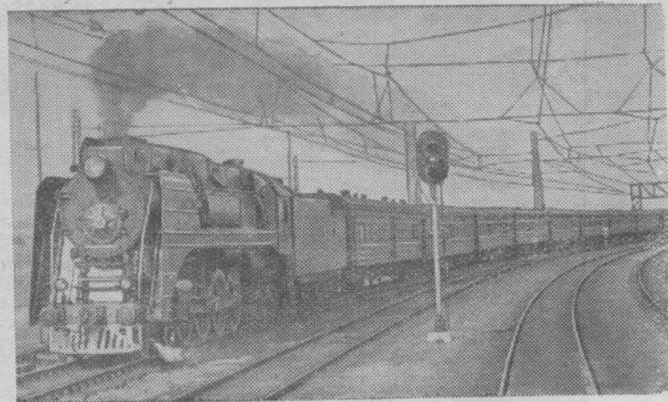
Москва. Коломенский паровозостроительный завод имени Куйбышева выпустил пассажирский паровоз типа „2-4-2“. Этот паровоз более экономичен в эксплуатации, чем другие пассажирские и товарные паровозы, может развивать скорость до 125 километров в час и водить тяжеловесные пассажирские поезда (до 18 вагонов).
