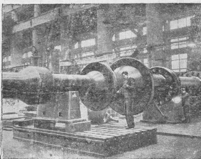
ЛЕНИНГРАД. В гидротурбинном цехе завода имени Сталина. Подготовка вала для очередной Днепровской турбины.
