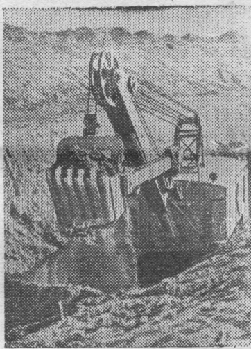
Красноярский край. В Канском угольном бассейне заканчивается строительство Ирша-Бородинского разреза.
