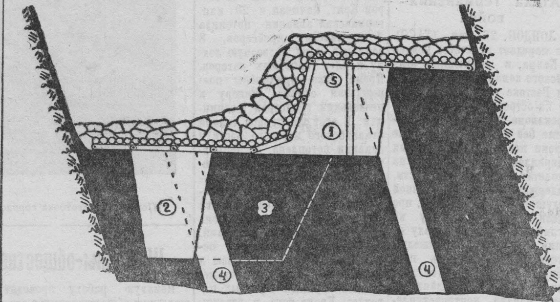
На снимке: общий вид железобалочного мата в работе (разрез вкrest простирания пласта). Условные обозначения: 1) призабойное пространство, 2) разрезной штрек нижнего слоя, 3) орта нижнего слоя, 4) углеспускные печи, 5) накатник.
