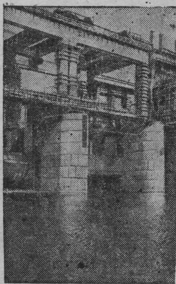
На строительстве Угличского гидроузла: вид на бычки плотины № 1 и железобетонную эстакаду после закрытия пролетов донными и шандорными щитами.
