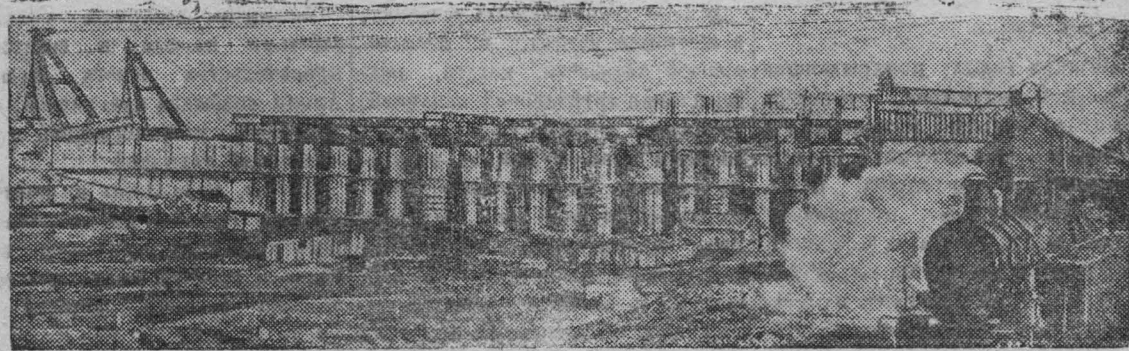
Панорама строительства Шекснинской ГЭС (мощность 330 тысяч киловатт). Фото М. Королева.
