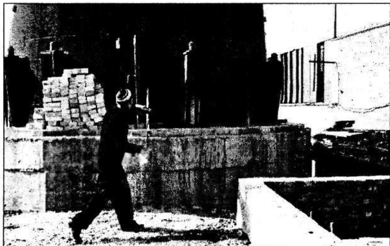
Перед пуском новой печи необходима сушка трубы. В ней разжигается костер, и через трое суток труба прогревается до 150 °С.
