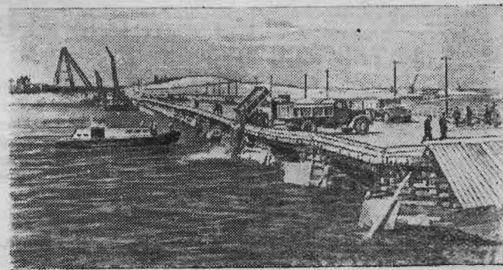
ГОРЬКОВСКАЯ ОБЛАСТЬ. Для перекрытия русла Волги на строительстве Горьковской гидроэлектростанции был сооружен понтонный мост шириной в 20 метров и длиной в 300 метров, с которого автосамосвалы сбрасывали камень.
