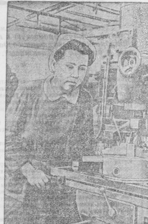
Сталинск. Кузнецкий машиностроительный завод выполняет заказы для великих строек коммунизма. На снимке: стахановка комсомолка Нина Москвина за изготовлением буровых коронок.
