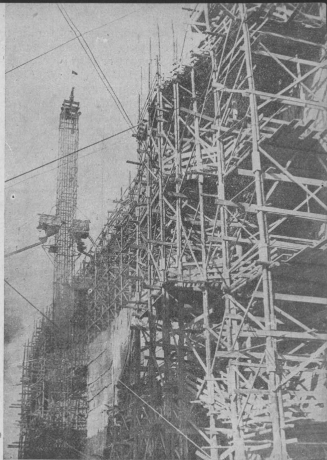
Магнитогорская центральная электростанция.
