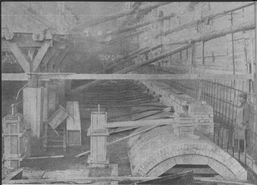
Консовый цех Кузнецкстроя. Укладка анкерных болтов 1-й батареи консовых печей (март 1931 г.)
