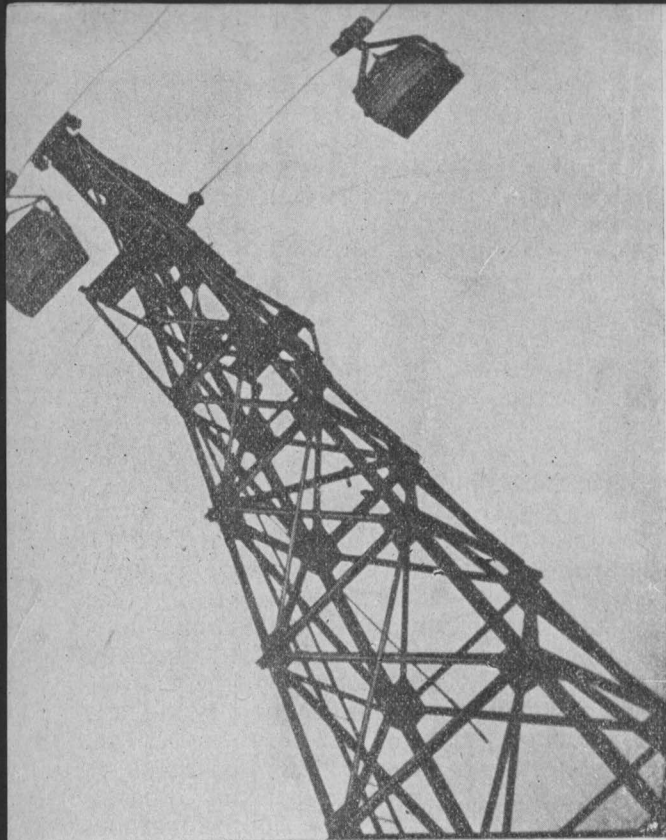
Кушвинский металлургический завод. Подача топлива в доменный цех по новой канатной дороге.
