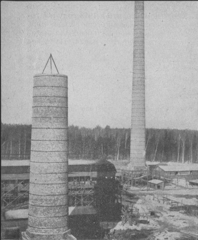
Красноуральский медеплавильный гигант. Самая высокая в СССР труба (105 метров).
