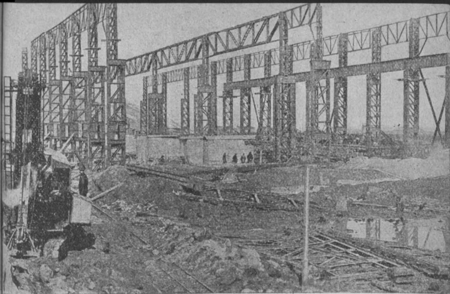
Мартеновский цех Кузнецкстроя в марте 1931 г. (установка колонн главного здания для первых семи печей).
