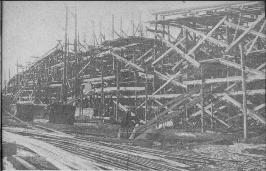
Литейный цех Кузнецистроя. Устройство лесов, арматуры и опалубки.
