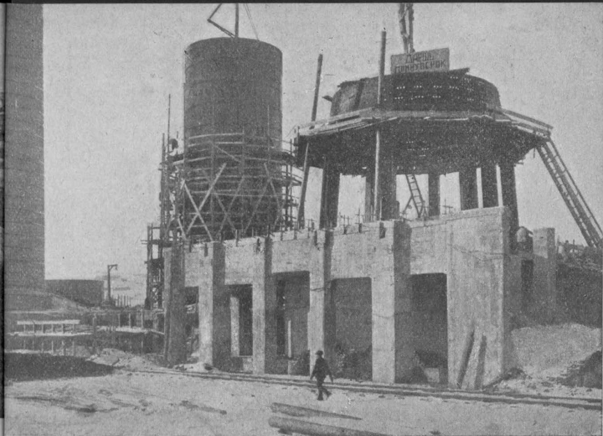
Доменный цех Кузнецкостроя в декабре 1930 г. (монтажные работы по домне и первому наперу).
