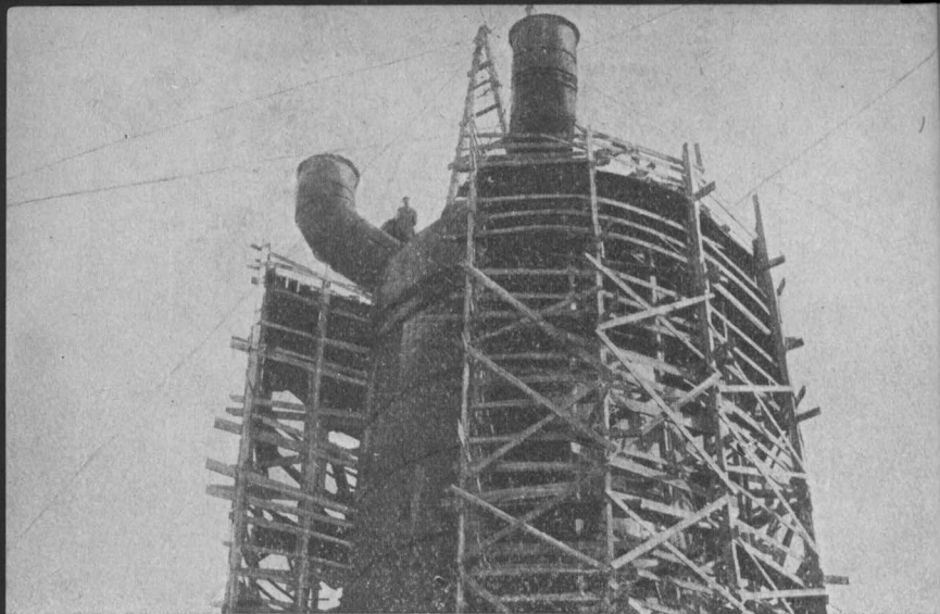
Доменный цех Кузнецкостроя в марте 1931 г. (монтаж газоотводов доменной печи № 1).
