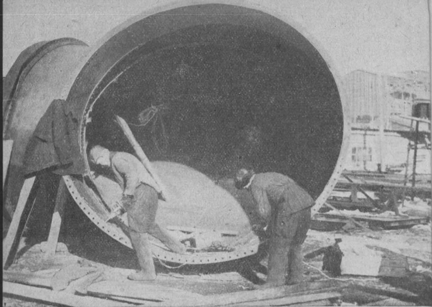
Уралмедьстрой. Клепка гигантской трубы для отвода воды [(март 1931 г.).
