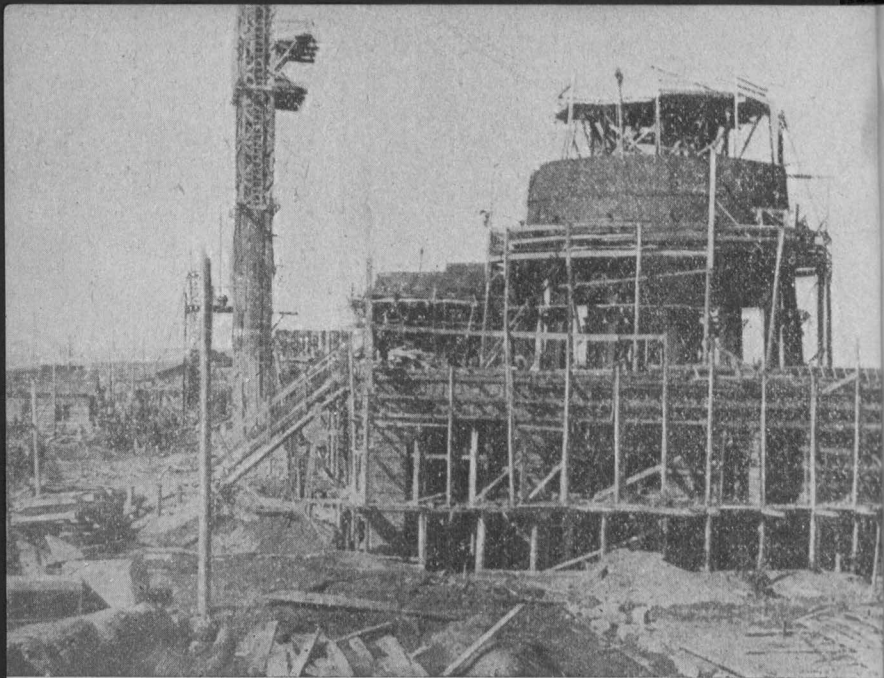
Монтаж домны № 1 на Магнитострое (май 1931 г.); готово два яруса.
