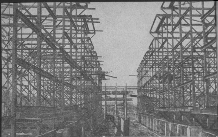
Магнитострой. Конструкции коксо-химического комбината (май 1931 г.)
