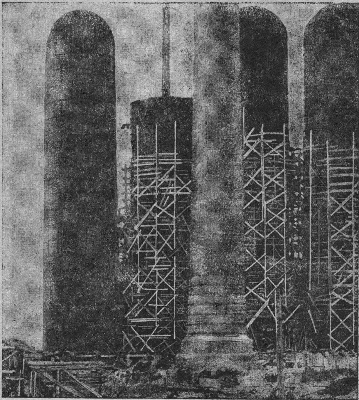
Сборка кауперов.
