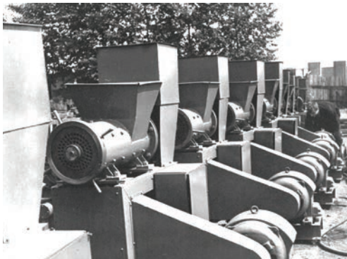
Корморезки – продукция завода «Строммашина» (1961 год)
